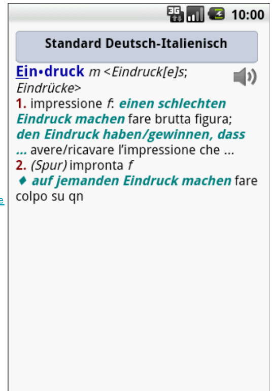
Vollbildschirm-Modus
